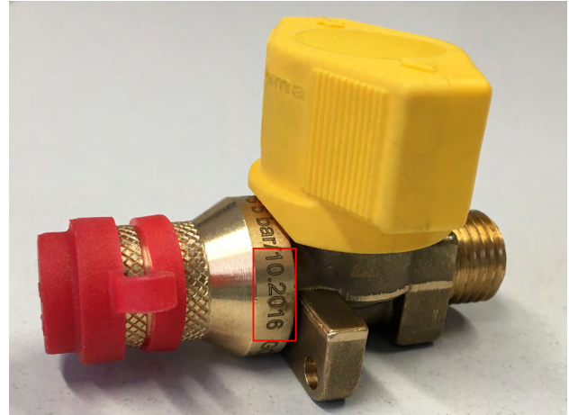
Codierung Beispiel 10.2016 (Ring zum Ablesen drehen)
